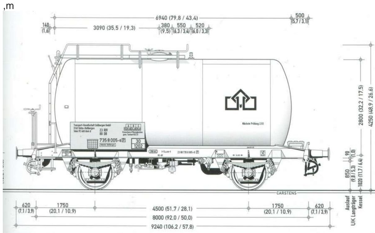
Bild 2: Vorbildskizze Leichtbau Kesselwagen Uerdingen- Quelle: St. Carstens, Güterwagen Bd. 7, Fürstenfeldbruck 2014
